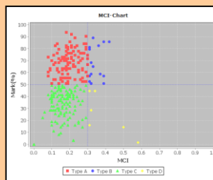
題目與受試者能力圖 (item-person map) 修正注意系數 (MCI)
