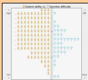
題目與受試者能力圖 (item-person map) 修正注意系數 (MCI)
